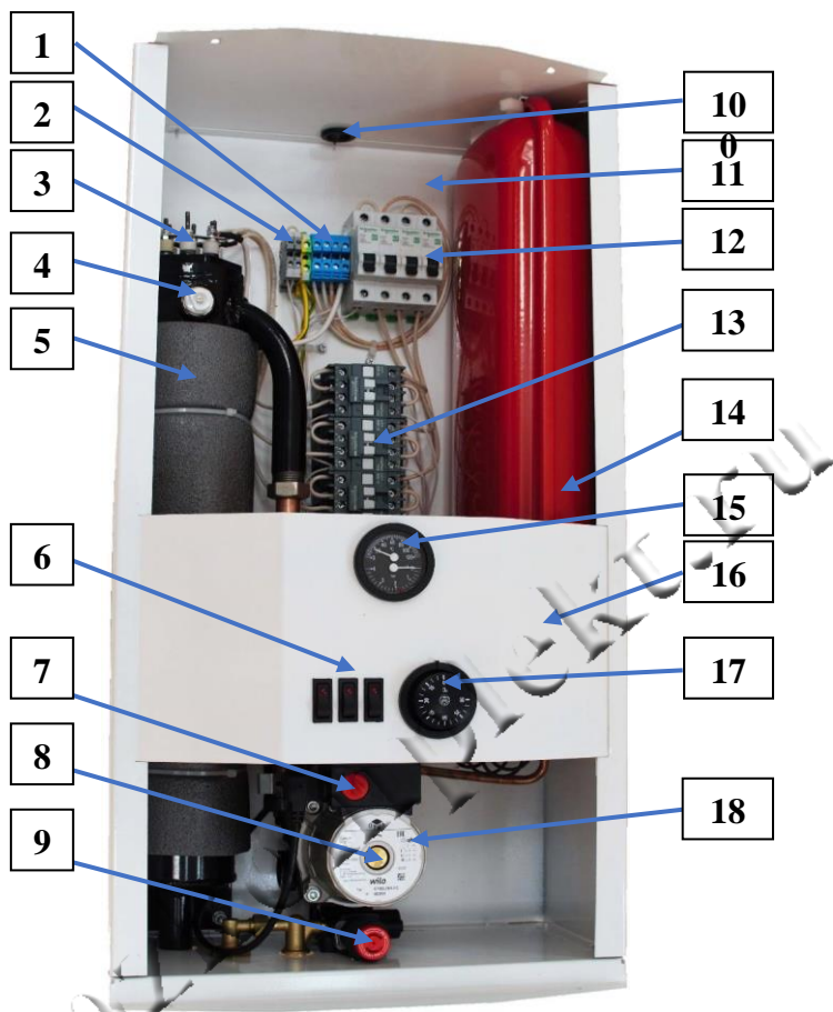
Рисунок 2. Электрокотел NEO со снятой лицевой панелью.
